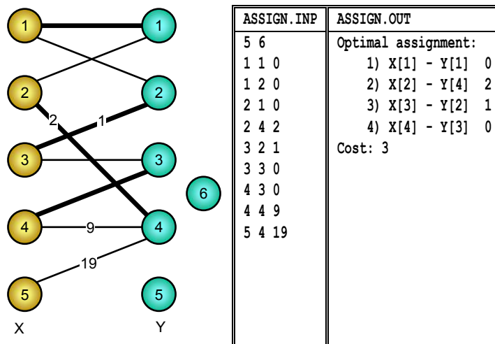
P_4_12_1.PAS * Thuật toán Hungari
